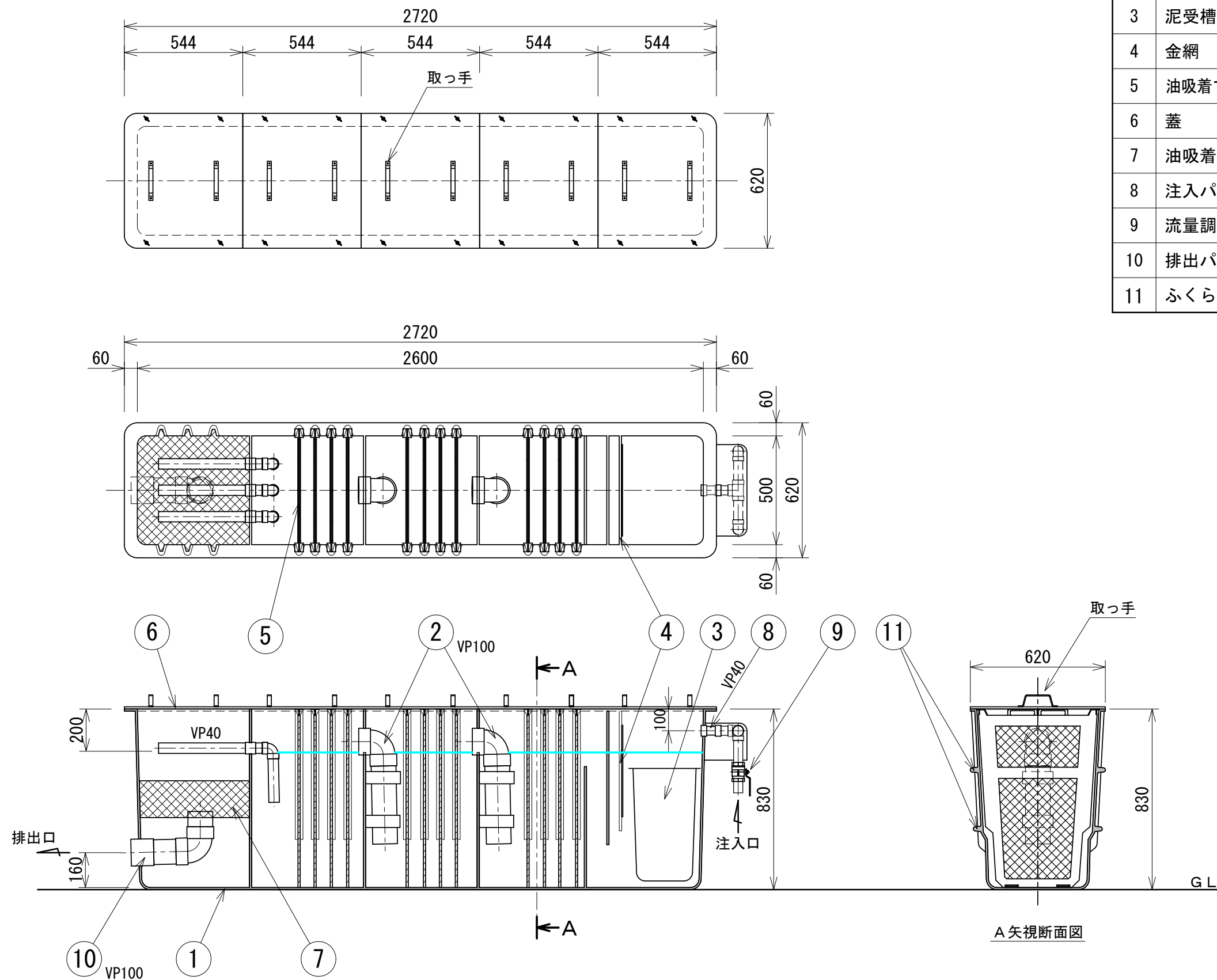
ワンタッチ交換式油吸着マット枠 12枚
